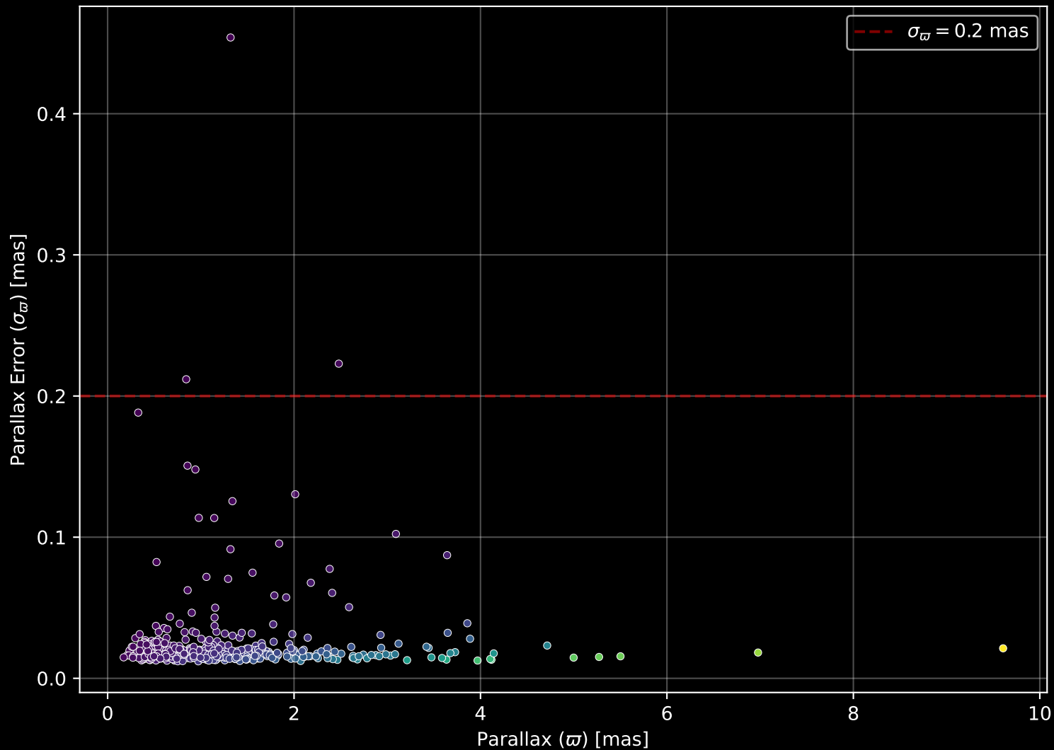
GALAH DR4 Field: [9394] Parallax Quality (n= 437)
