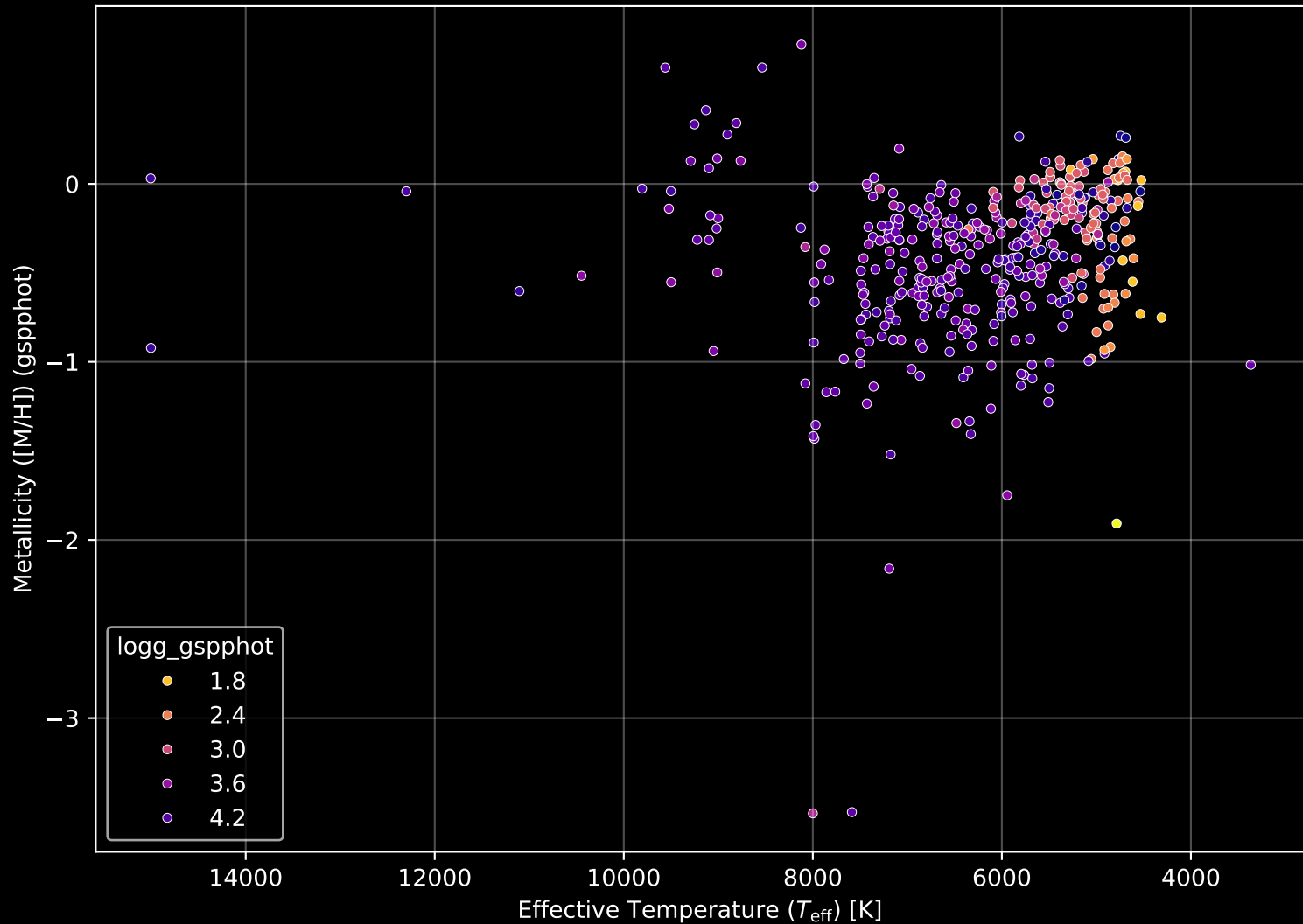
GALAH DR4 Field: [9394] Stellar Population Parameters (n= 437)
