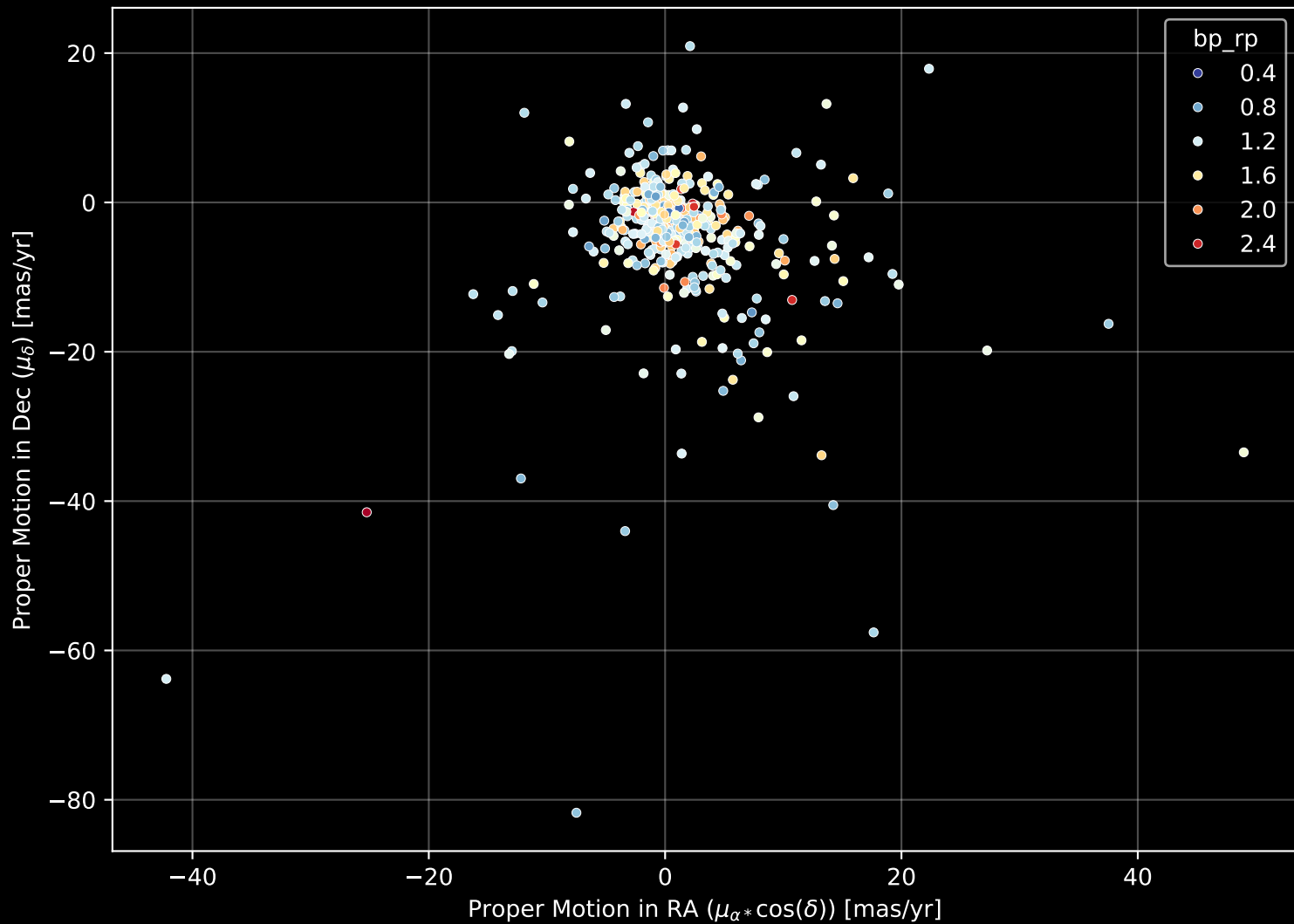
GALAH DR4 Field: [9394] Proper Motion Diagram (n= 437)
