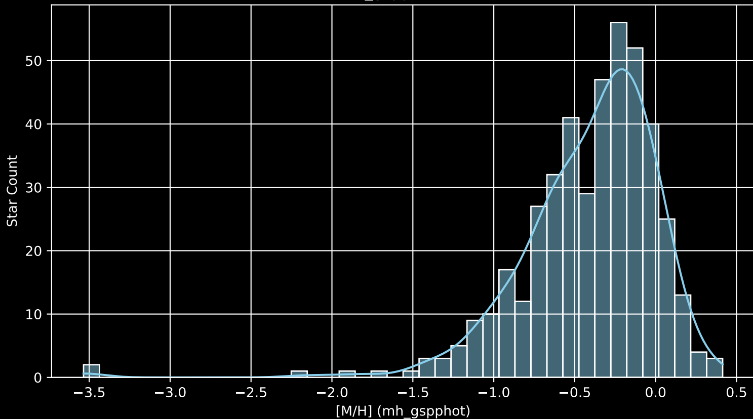
GALAH DR4 Field: [9394] [M/H] (mh_gspphot) (n= 434)
