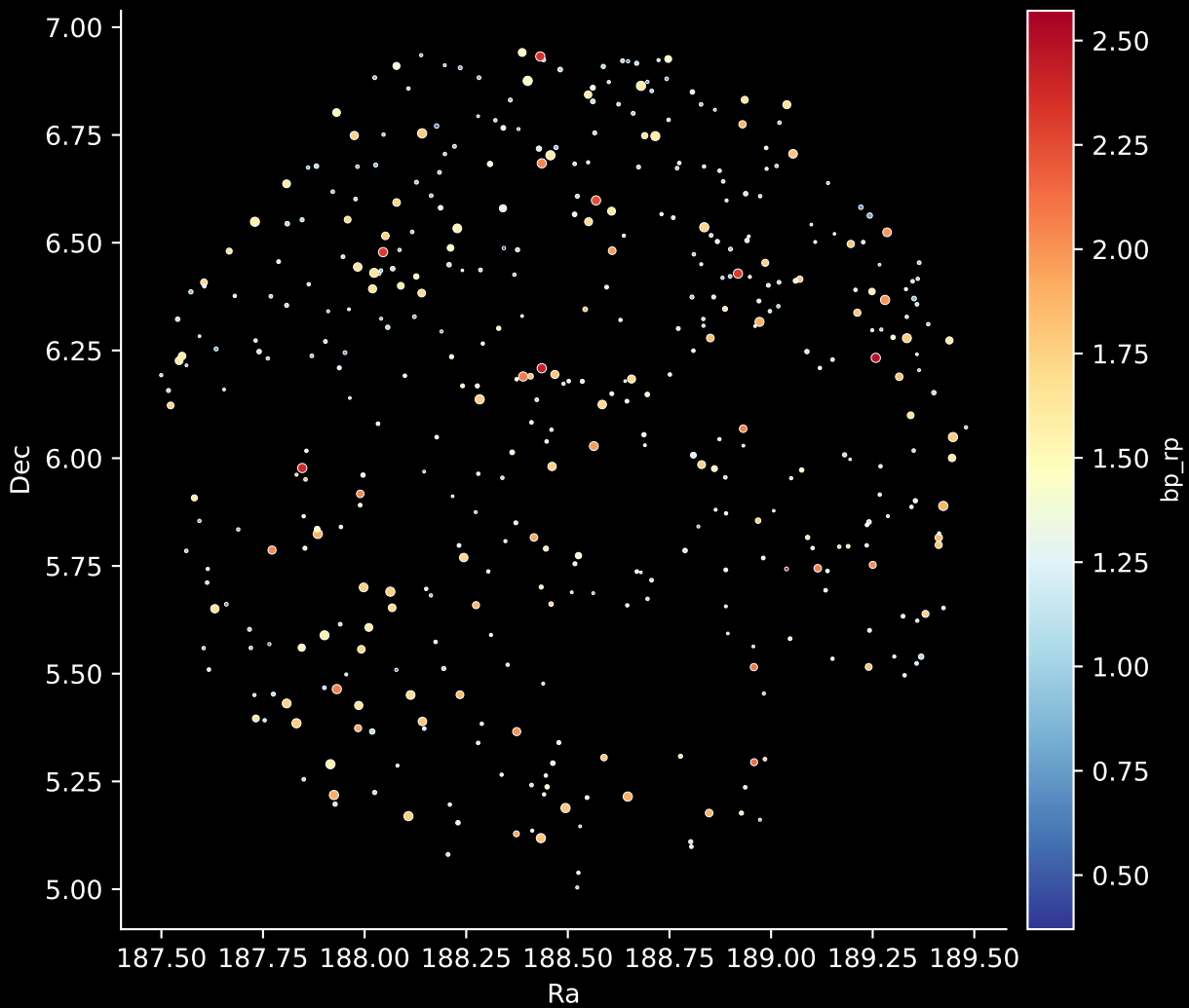
GALAH DR4 Field: [9394] Stars: 437
